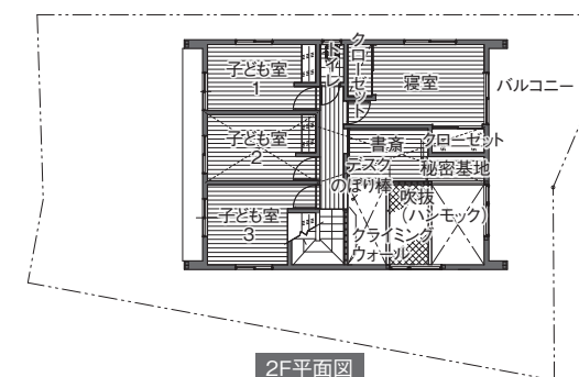
2F平面図
