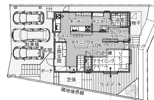
1F平面図
